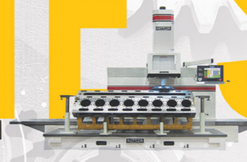
ХӨДӨЛГҮҮР СЭРГЭЭН ЗАСВАРЛАГЧ BORING SURFACE MACHINE
